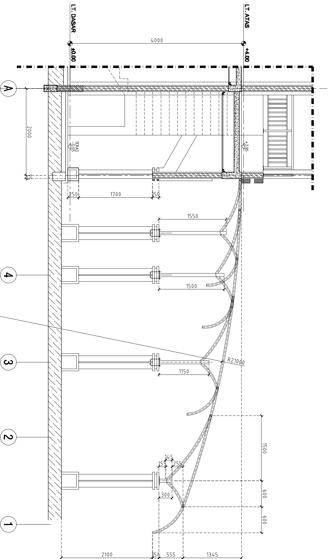
1 POTONGAN A-A CANOPY TERAS SKALA 1 : 50
